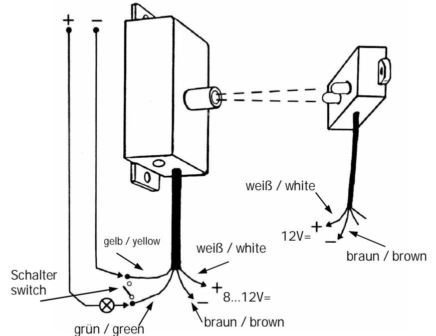
Anschlußbeispiel für eine Lampe Connecting example for lamp
