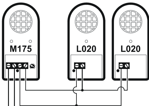
12 V/DC Anschlussmöglichkeit für 2 Zusatzlautsprecher L020 Possibility to connect 2 additional loudspeakers L020
